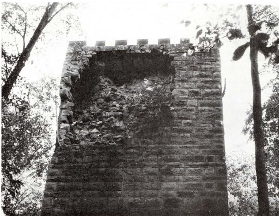
Abb. 1. Rötterturm vor der Sanierung, 1972
