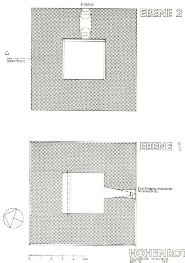
Abb. 4. Röterturm. Grundrisse, September 1972
