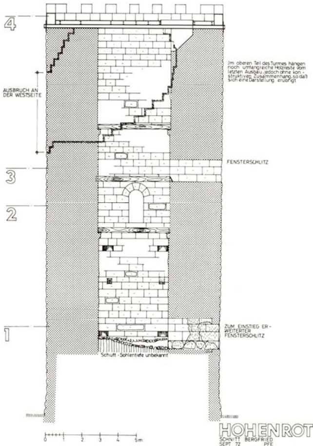
Abb. 3. Röterturm, Schnitt, September 1972
