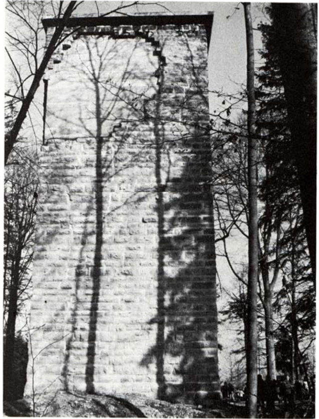
Abb. 2. Röterturm nach der Sanierung, 1974
